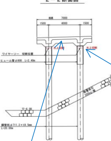
2-2断面図
