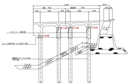
1-1断面図
