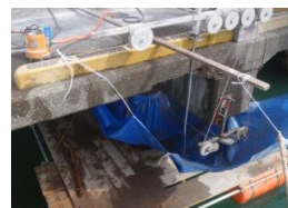
ワイヤーソー切断工
